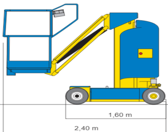
2.5.1 - Encombrement pour le mât ORION 1000
